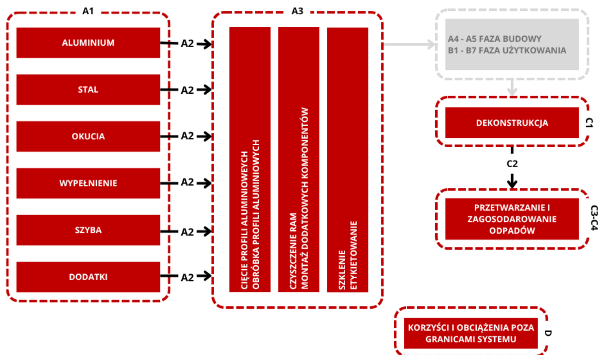
Rysunek 5.1: Granice systemu dla charakterystyki środowiskowej
